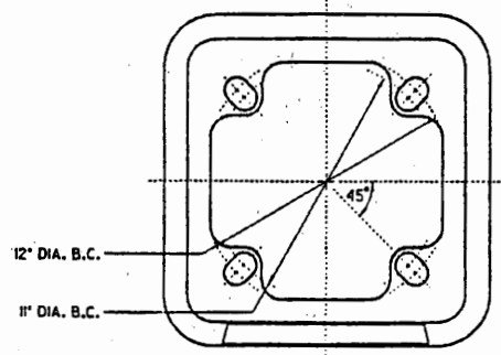
TOP VIEW N.T.S.
