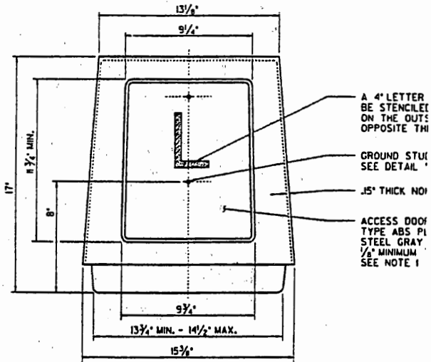
ELEVATION N.T.S.
