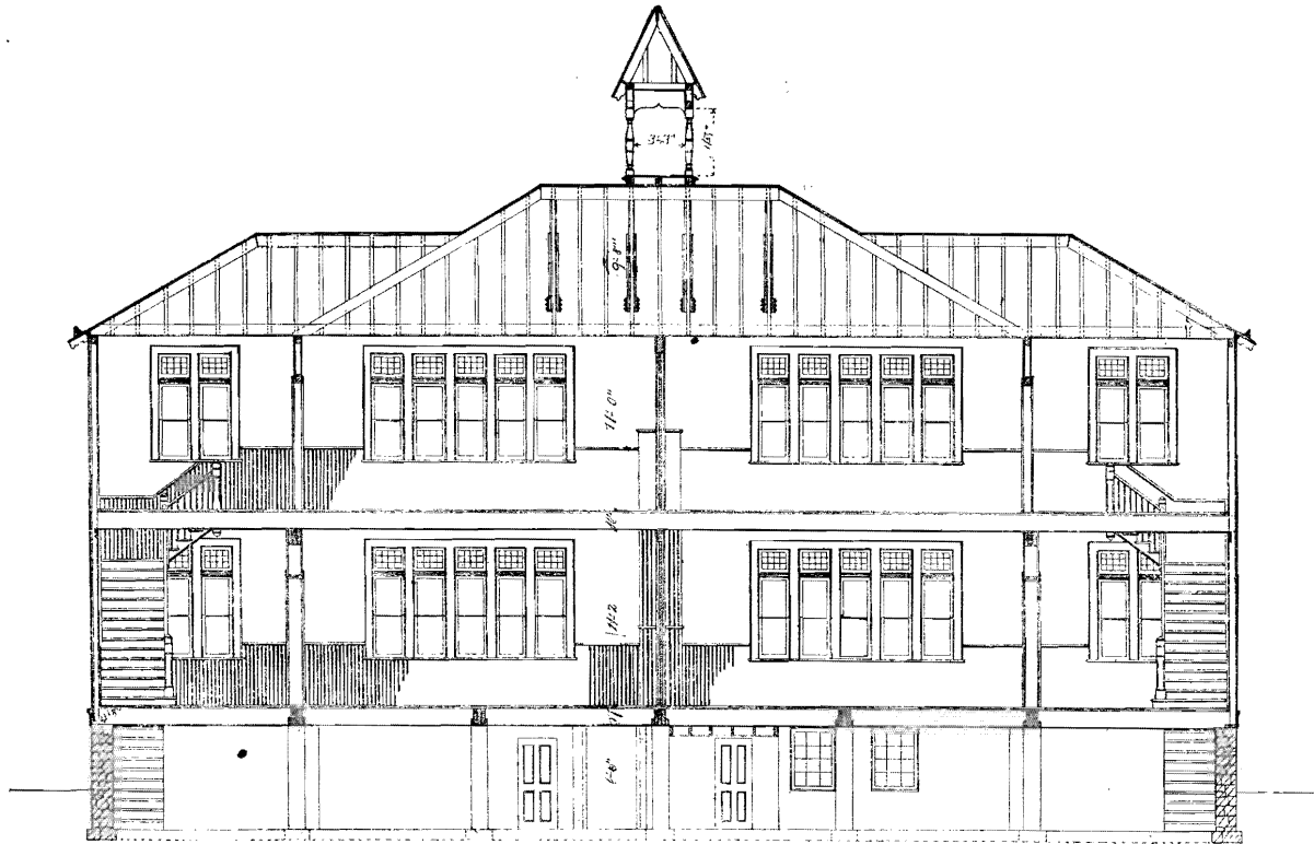
LONGITUDINAL SECTION.
